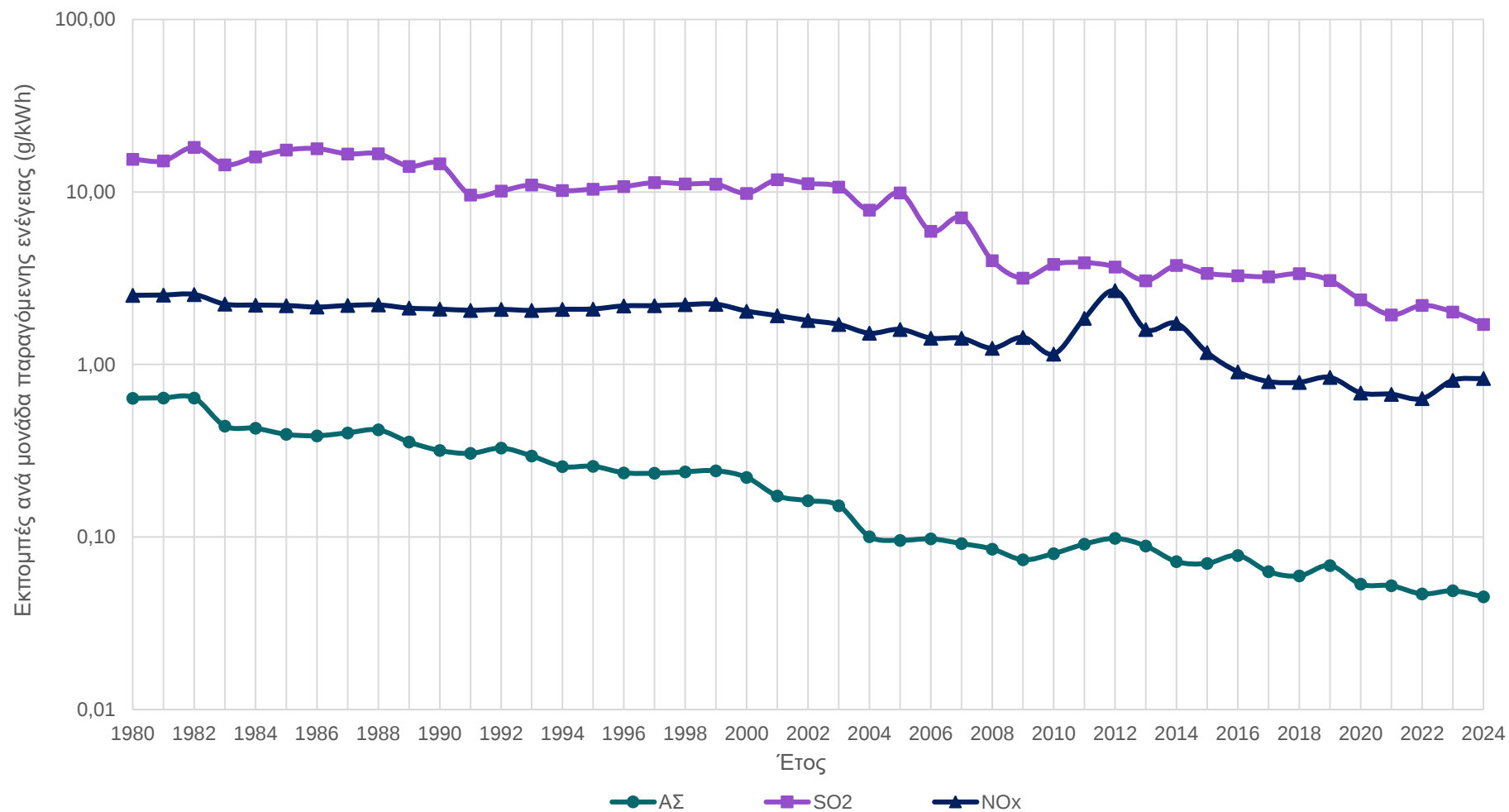
Γράφημα - Ετήσια διακύμανση περιβαλλοντικών δεικτών εκπομπών ΑΣ, SO 2 , NO x σε γραμμάρια ανά κιλοβατώρα από συμβατικές μονάδες ηλεκτροπαραγωγής μεγάλης κλίμακας (λογαριθμική κλίμακα)
